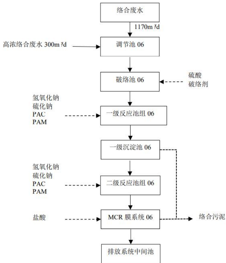
图 7.1-4 浓络合废水处理流程图
