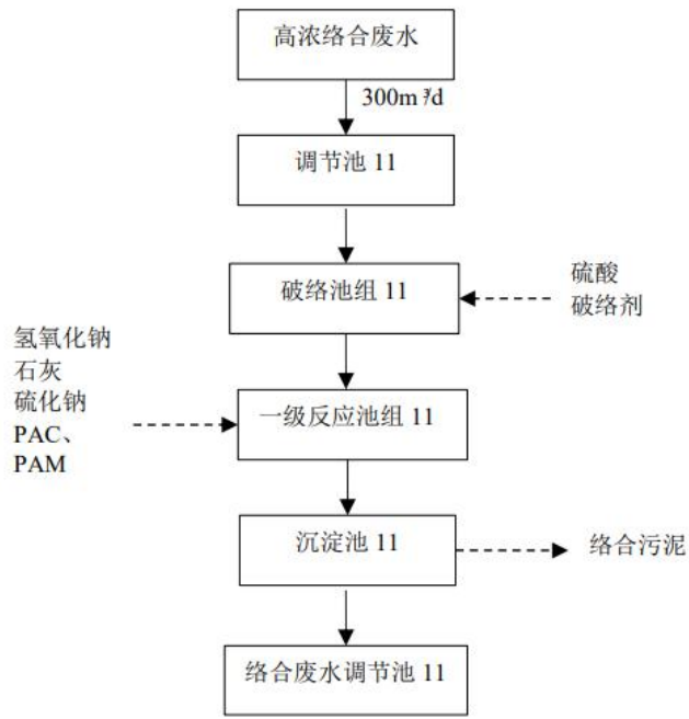
图 7.1-3 高浓络合废水处理流程图
