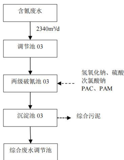
图 7.1-5 含氰废水处理流程图
